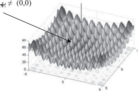
شکل ۱: مفهوم بهینه‌های محلی و بهینه جامع
