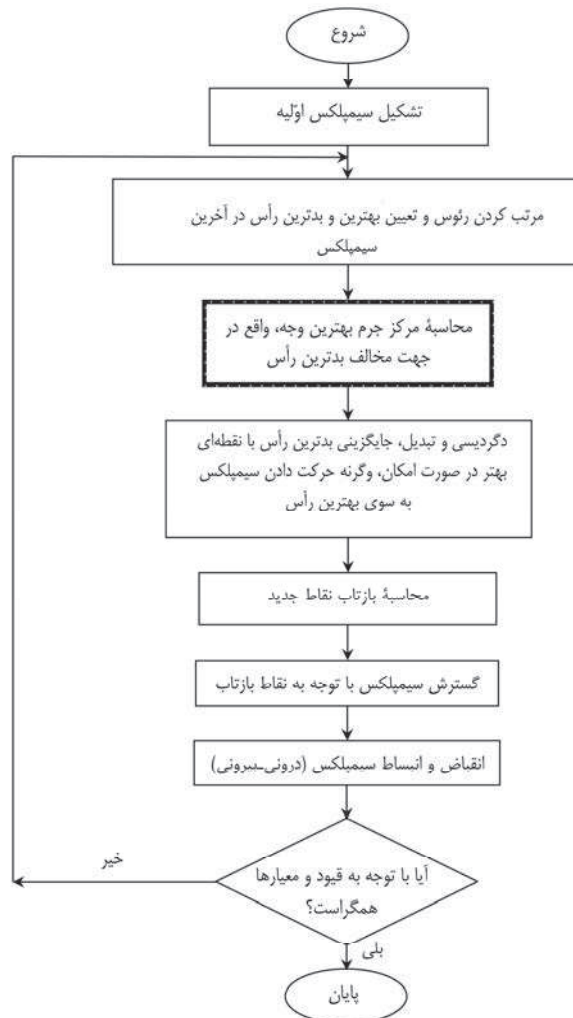
شکل ۴: فلوجارت الگوریتم نلدر - مید (منبع: اقتباس مؤلف‌ها از الگوریتم نلدر - مید)
